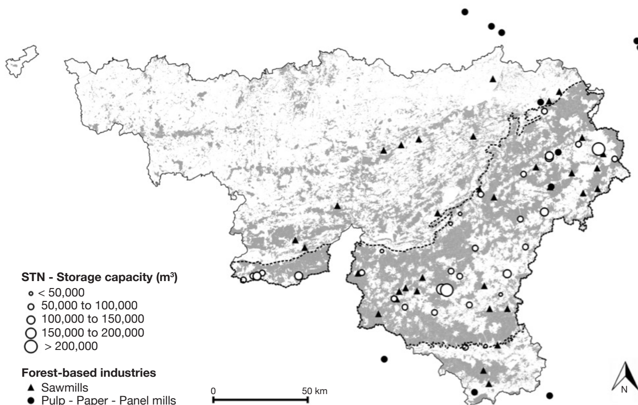
Figure 7. Suggested locations of a sprinkling storage terminals network (STN) in Wallonia and proximity to forest-based industries — Localisation potentielle d'un réseau de sites de stockage (STN) de bois sous aspersion en Wallonie et proximité des industries de la filière bois.
