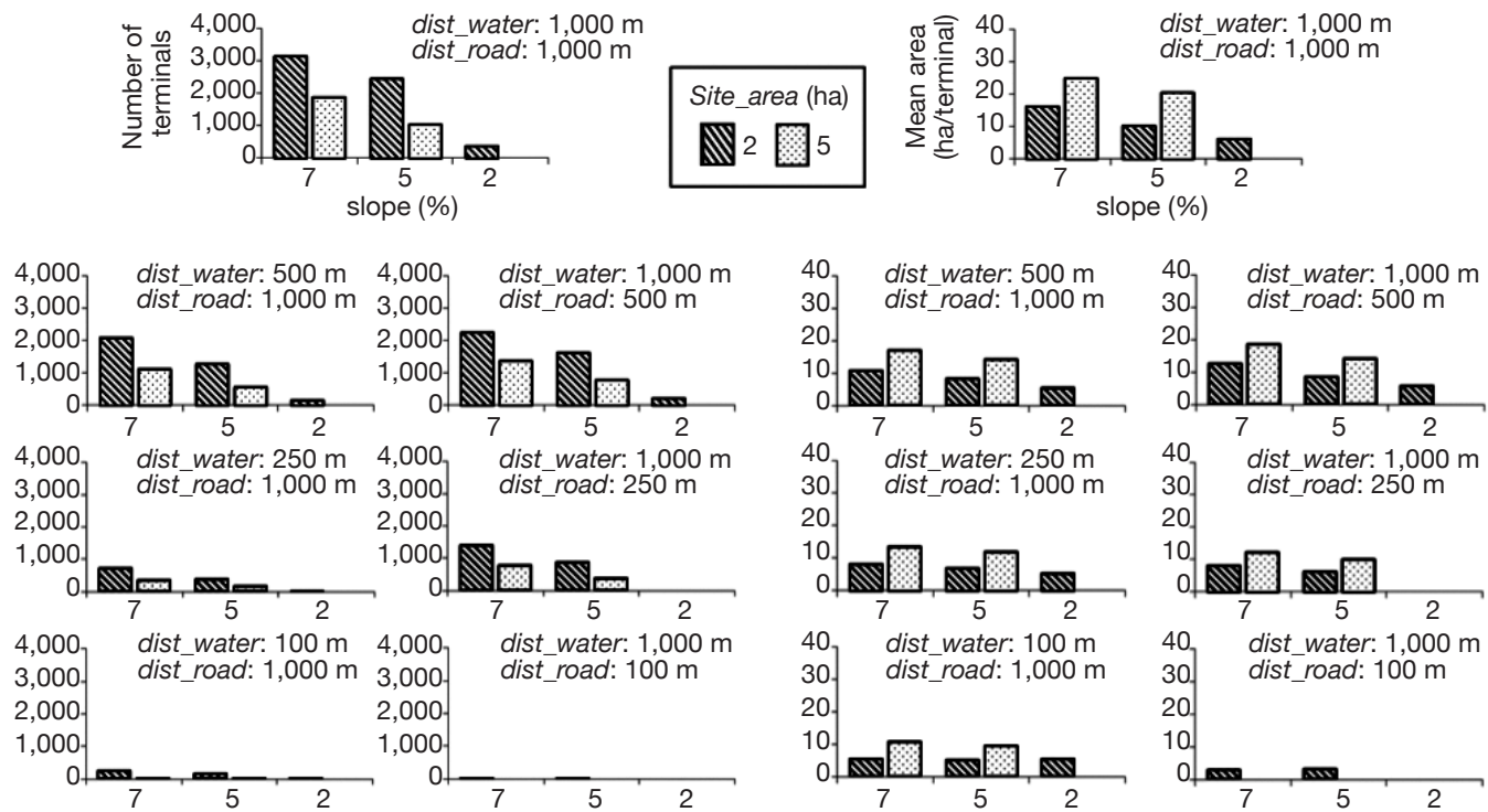
Figure 6. Influence of criteria ( slope\_max , site\_area , dist\_wate , dist\_road ) on the results in terms of number and size of sprinkling storage terminals — Influence des critères de sélection des sites ( slope\_max , site\_area , dist\_wate , dist\_road ) sur les scénarios en termes de nombre et de superficie.
